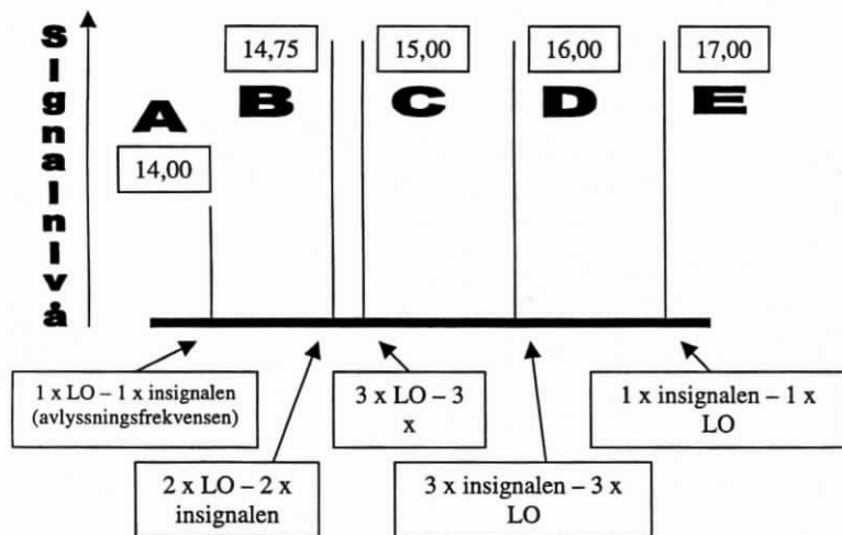
Fig 4, frekvensspektra med önskade och oönskade signaler
