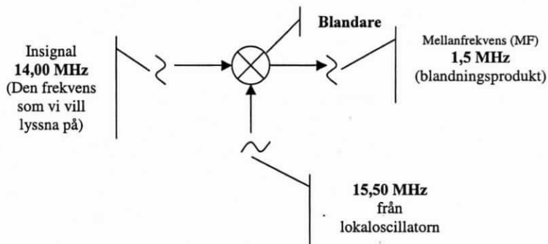
Fig 3, Blandarens arbetssätt
