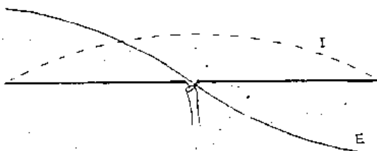
Ström- och spänningfördelning på en halv vågsdipol.
